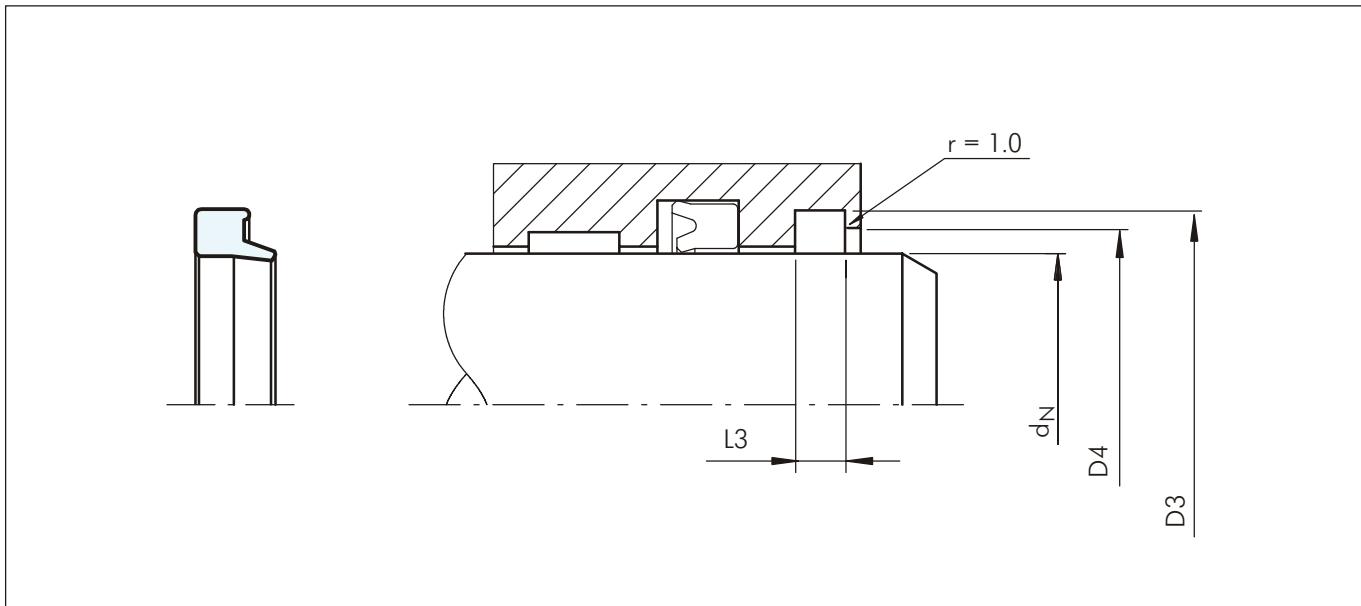
Рисунок 18 Схема монтажа
