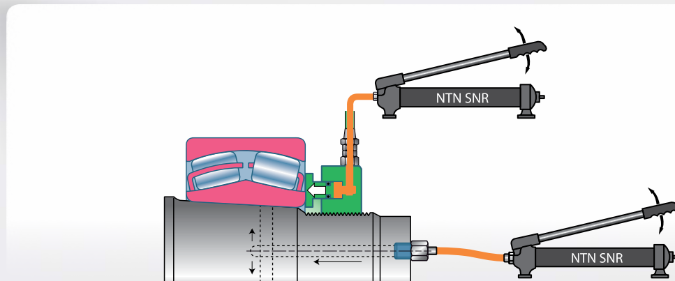
Одновременное использование гидравлической гайки и впрыска масла для создания масляной пленки
